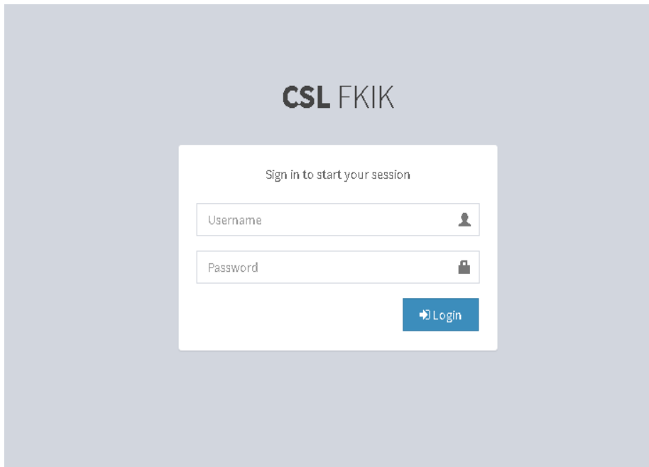
Gambar 1. Tampilan awal
